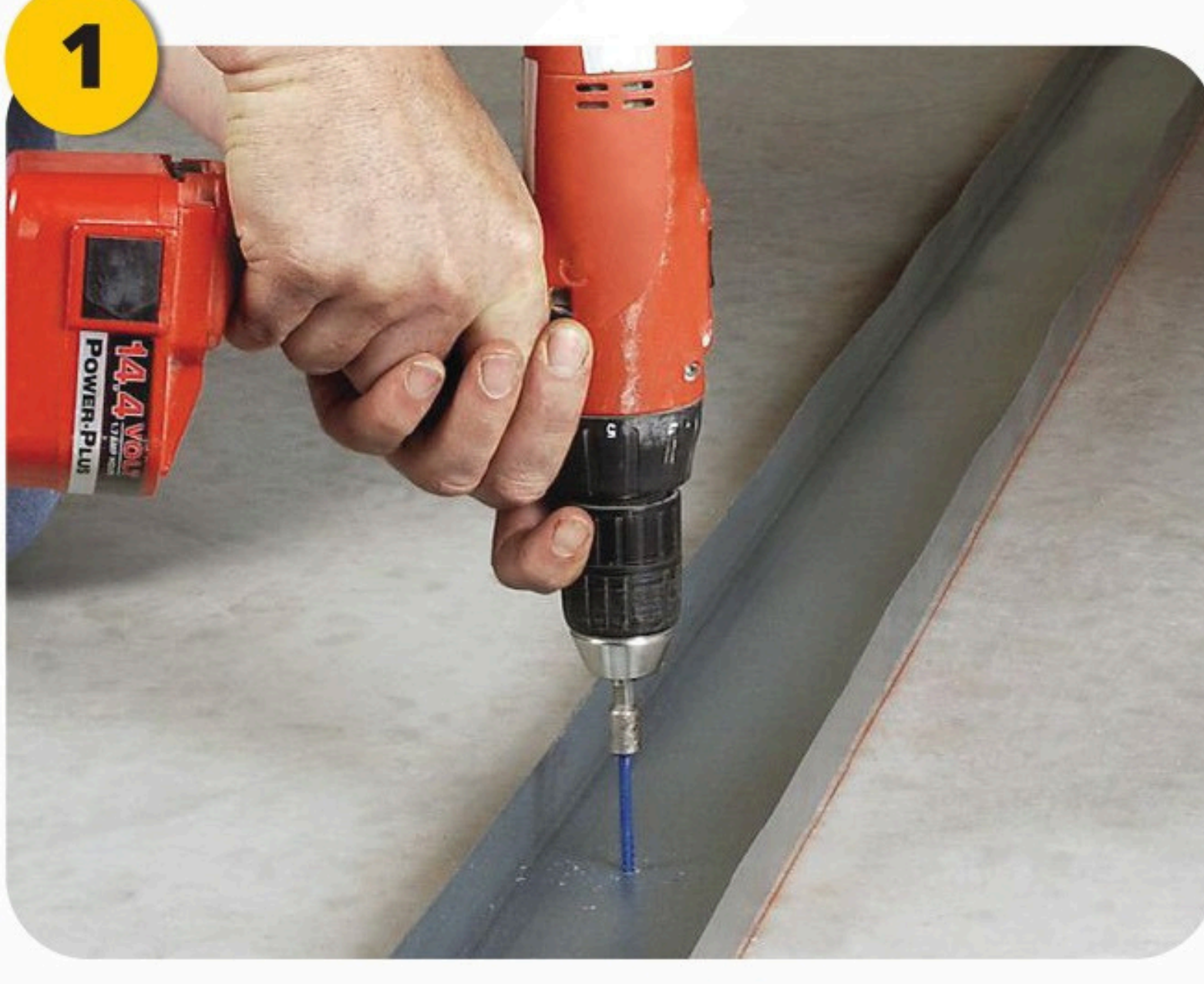
1 சீலிங் மற்றும் தரை சேனல்களை பொருத்தவும்
