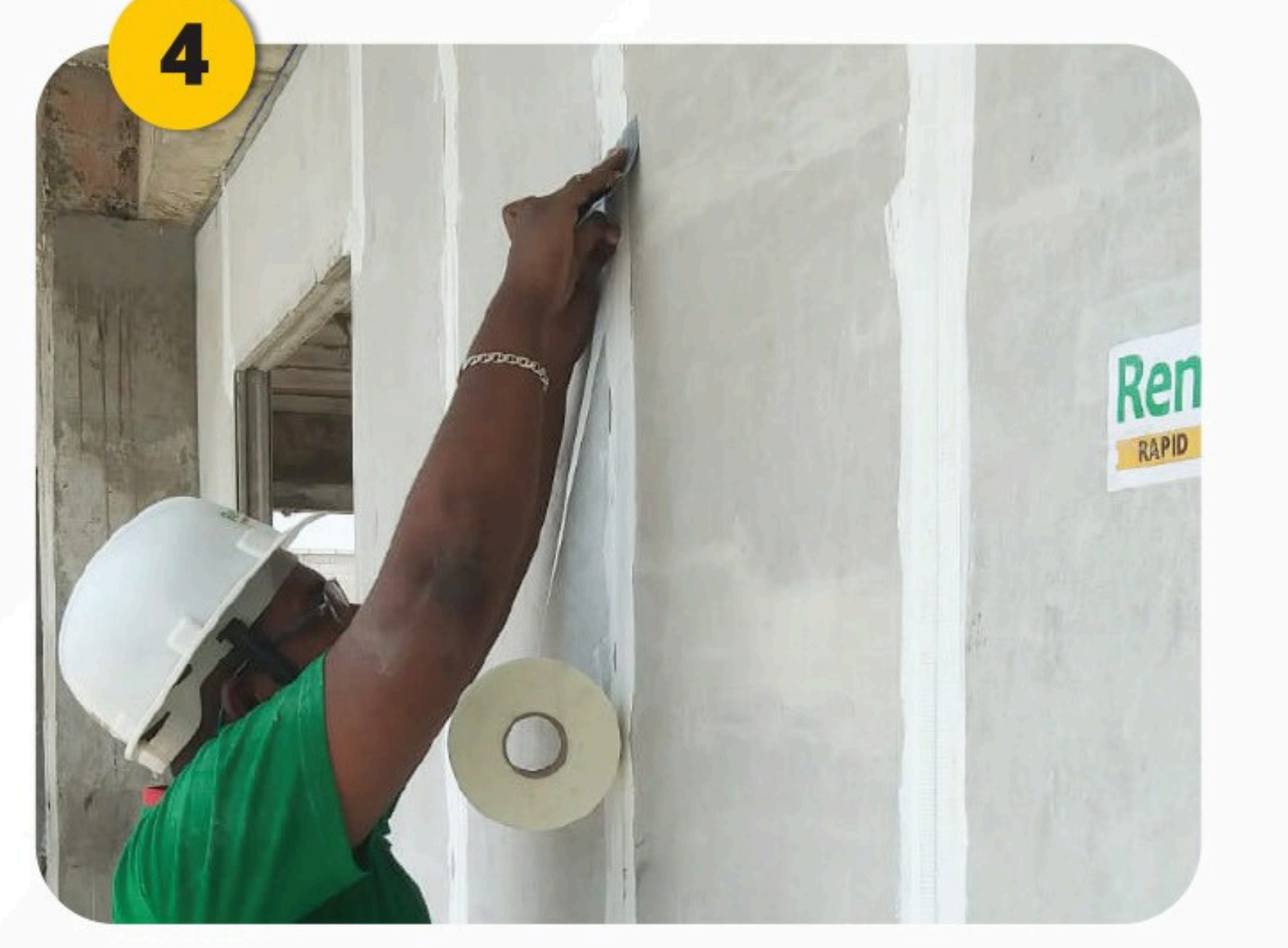
4 TONGUE AND GROOVE JOINT - ல் FIBER MESH - ஐ ஒட்டவும்
